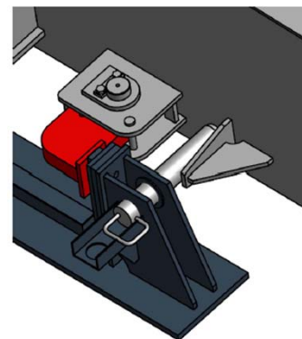
■ End stopper 端部限位
