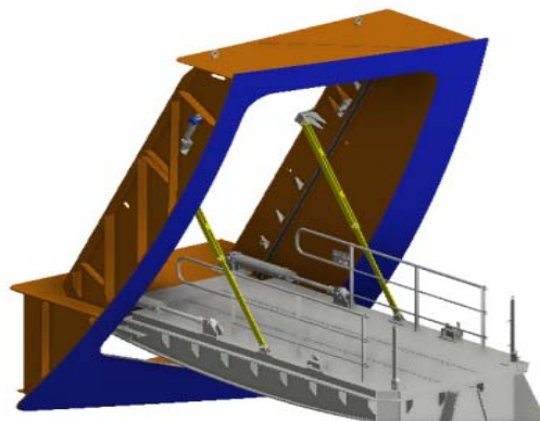
■ Observation Platform 观测台
