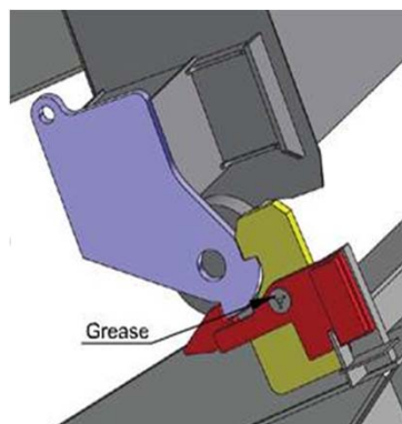
■ End stopper 端部限位
